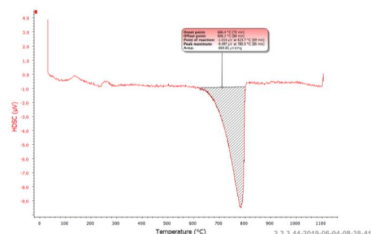
Рис.3. HDSC кривая известняка Уч-Учакского месторождения
