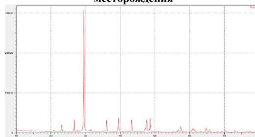
Рис.4. Рентгенограмма известняка Уч-Учакского месторождения
